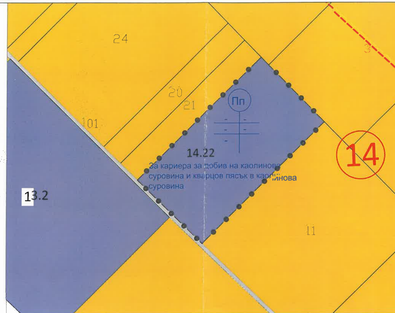
ПУП - ПЛАН ЗА ЗАСТРОЯВАНЕ ЗА ПИ 66229.14.22 ПО КККР НА гр.СЕНОВО общ.ВЕТОВО
